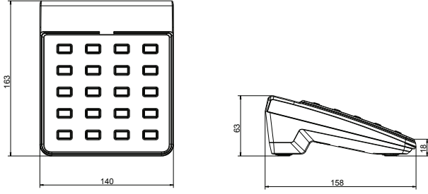
Şek. 1: Boyutlar
